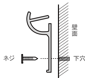
①ネジ による直付け
