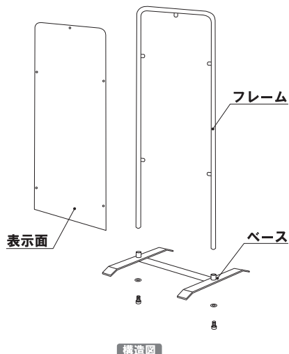
構造図
