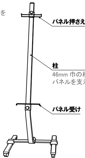
構造図
