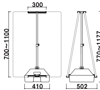
PG32R-B1との組み合わせ例
